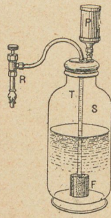
Sifón-filtro
