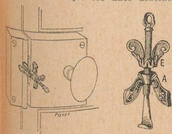
Figs. 3 y 4. Cerrojo Ideal
